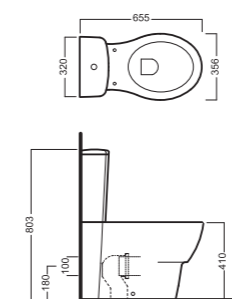
NIDO унитаз Моноблок
