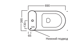
MARILYN унитаз Моноблок
