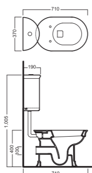
DOLCEVITA унитаз напольный с бачком
