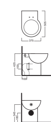
YOU & ME унитаз напольный угловой, правый Устанавливается с встроенным бачком (YXDX)
