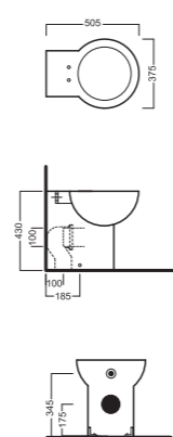
YOU & ME унитаз напольный с сиденьем Устанавливается с встроенным бачком (YXDX)
